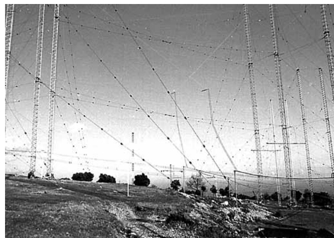
Jedno z anténních „hnízd“ na vršku hory nad Monte Carlem. Takových systémů je na kopci několik a každý je směřován do jiné části světa.
